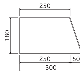
側面図 Scale1/10
