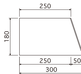
側面図 Scale1/10
