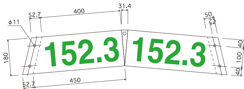
展開図 Scale1/10
